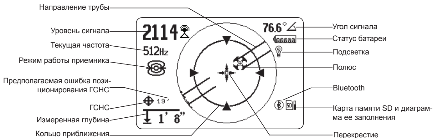
Рисунок 2 – Пример дисплея режима Зонд
